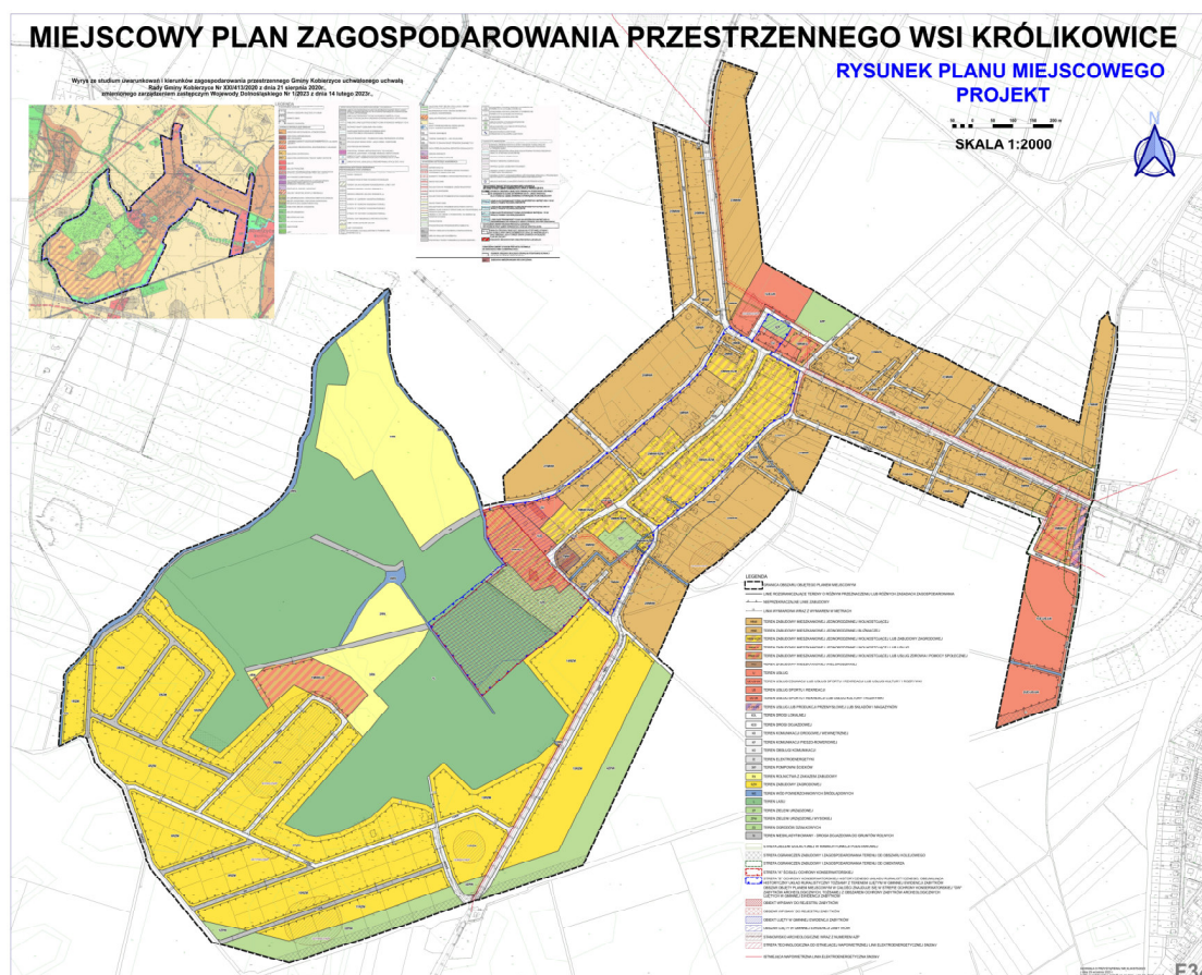
Ryc. 1 Rysunek projektu miejscowego planu zagospodarowania przestrzennego wsi Królikowice (źródło: opracowanie własne)
